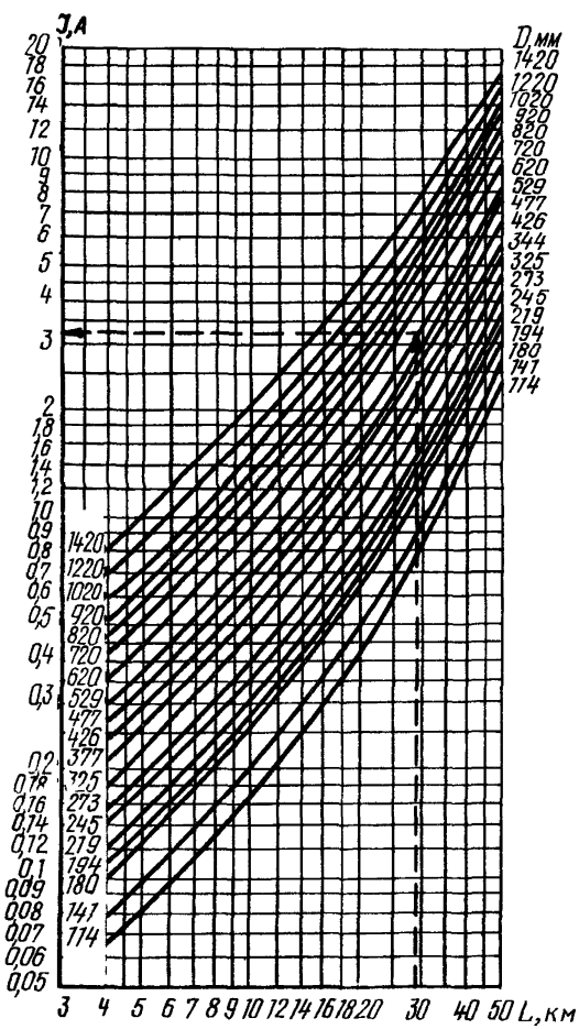
Рис.6. Номограмма определения силы тока для участков трубопровода длиной 4–50 км; изоляция из полимерных материалов (пример пользования номограммой для участка длиной 29 км диаметром 520 мм, сила тока при контроле I = 3,2 А)
