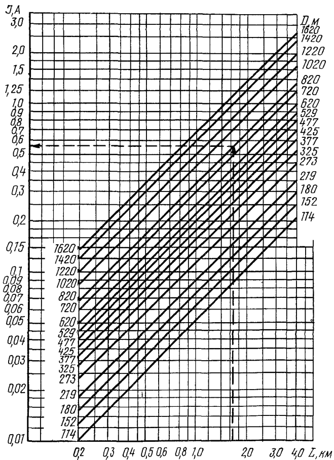
Рис.7. Номограмма определения силы тока для участков трубопровода длиной 0,2–4 км, изоляция на битумной основе (пример пользования номограммой для участка длиной 1,65 км, диаметром 820 мм, сила тока при контроле I = 0,56 А)
