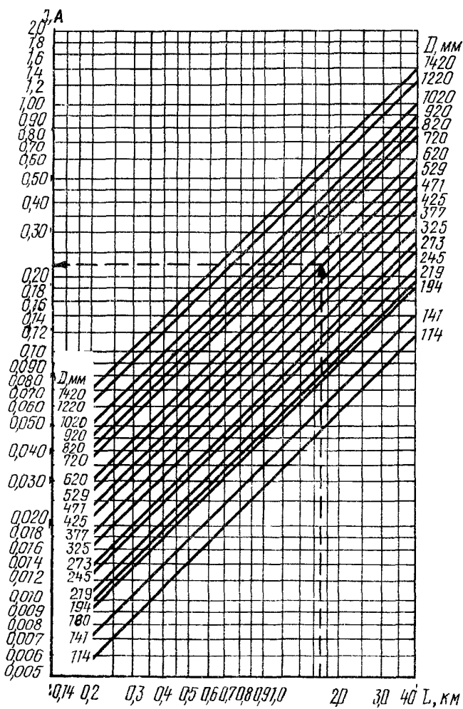
Рис. 8. Номограмма определения силы тока для участков трубопровода длиной 0,2–4 км, изоляция из полимерных материалов (пример пользования номограммой для участка длиной 1,7 км, диаметром 529 мм, сила тока при контроле J = J_{2,3} А)
