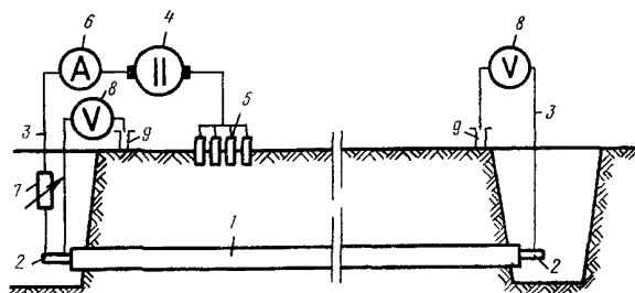
Рис. 3. Принципиальная схема подключения источника тока и измерительных приборов к контролируемому участку:
